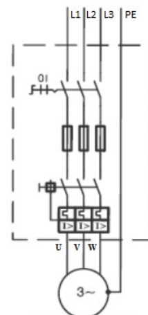
Schemat elektryczny podłączenia pomp 3-fazowych
