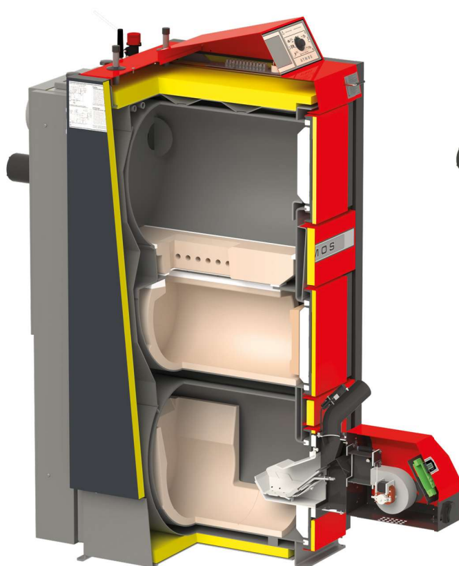
DC 18 SP, DC 25 SP, DC 30 SPX, DC 32 SP DŘEVO + PELETY
