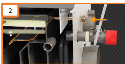
Zatápěcí klapka otevřena
