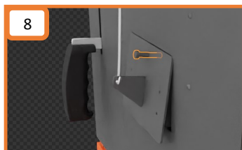
8 Minimální otevření primární klapky - klapka nesmí být nikdy úplně zavřena
