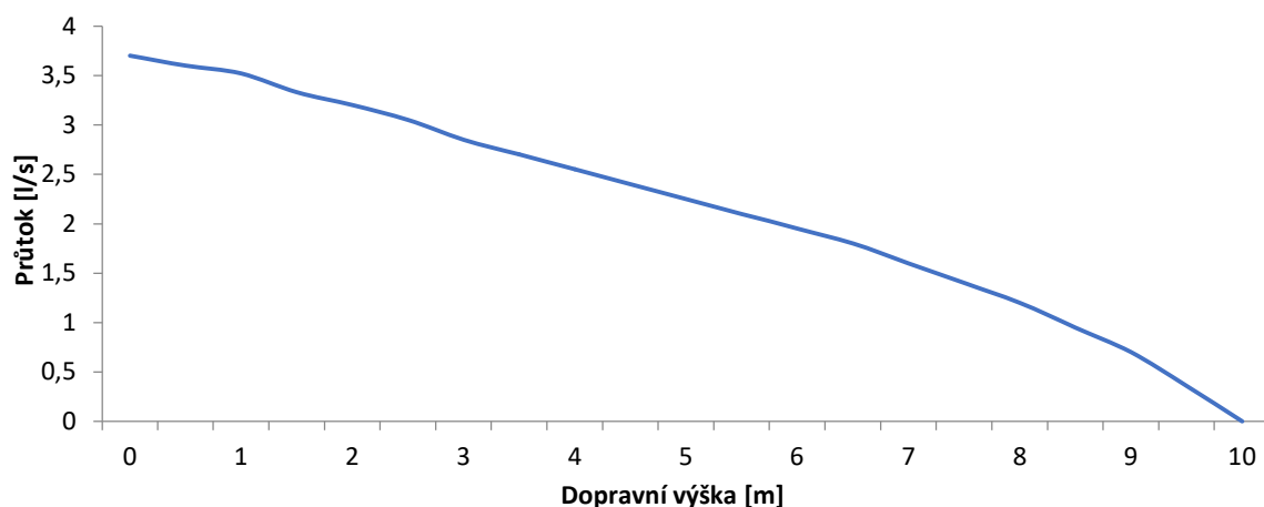
Q-H charakteristika pro čerpadlo PCH K1-J-220
